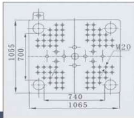
模板正面尺寸 Platen Dimensions
