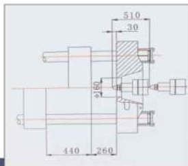
模板側面尺寸 Platen Dimensions
